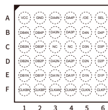
FO-36L
